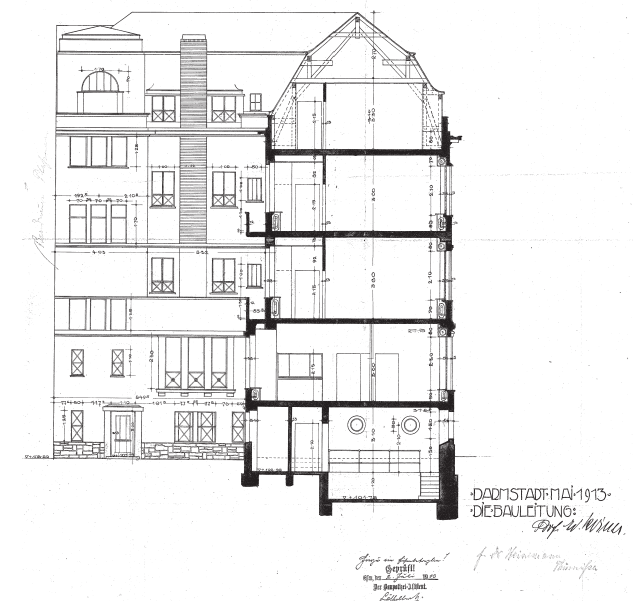
Schnitt A – B
